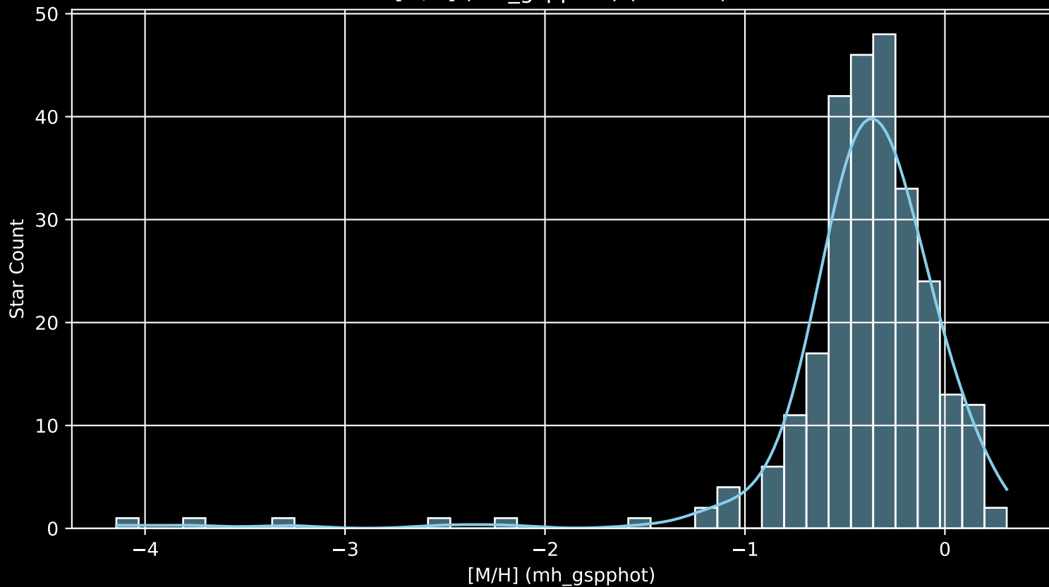
GALAH DR4 Field: [8686] [M/H] (mh_gspphot) (n= 266)
