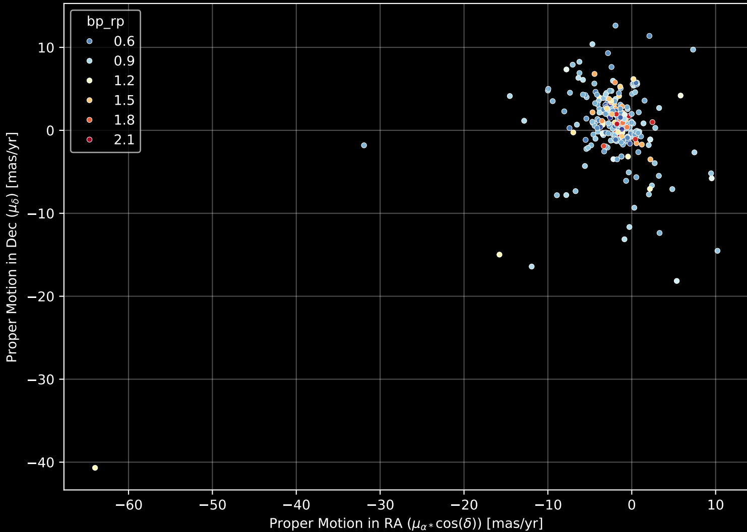
GALAH DR4 Field: [8686] Proper Motion Diagram (n= 266)
