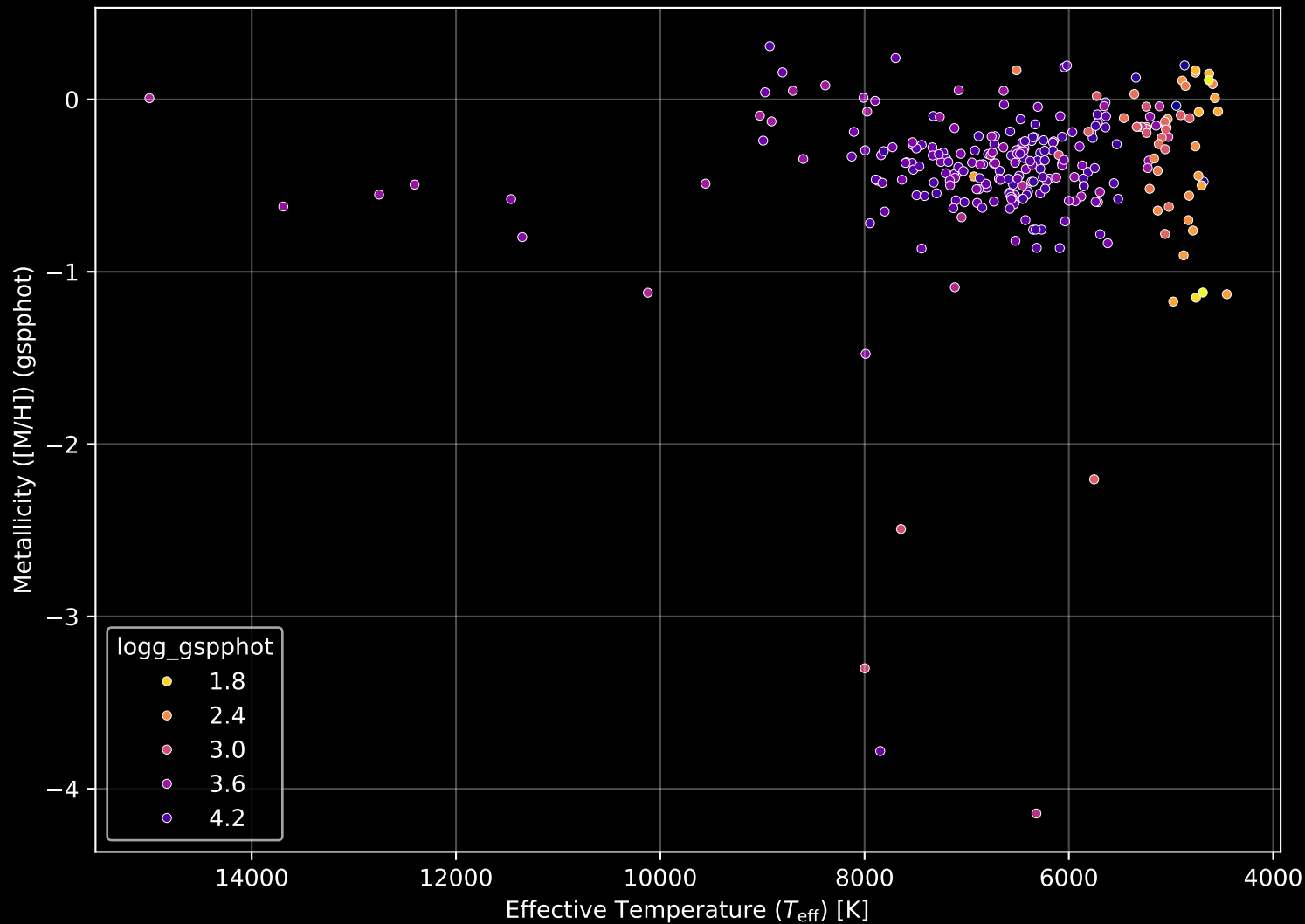
GALAH DR4 Field: [8686] Stellar Population Parameters (n= 266)
