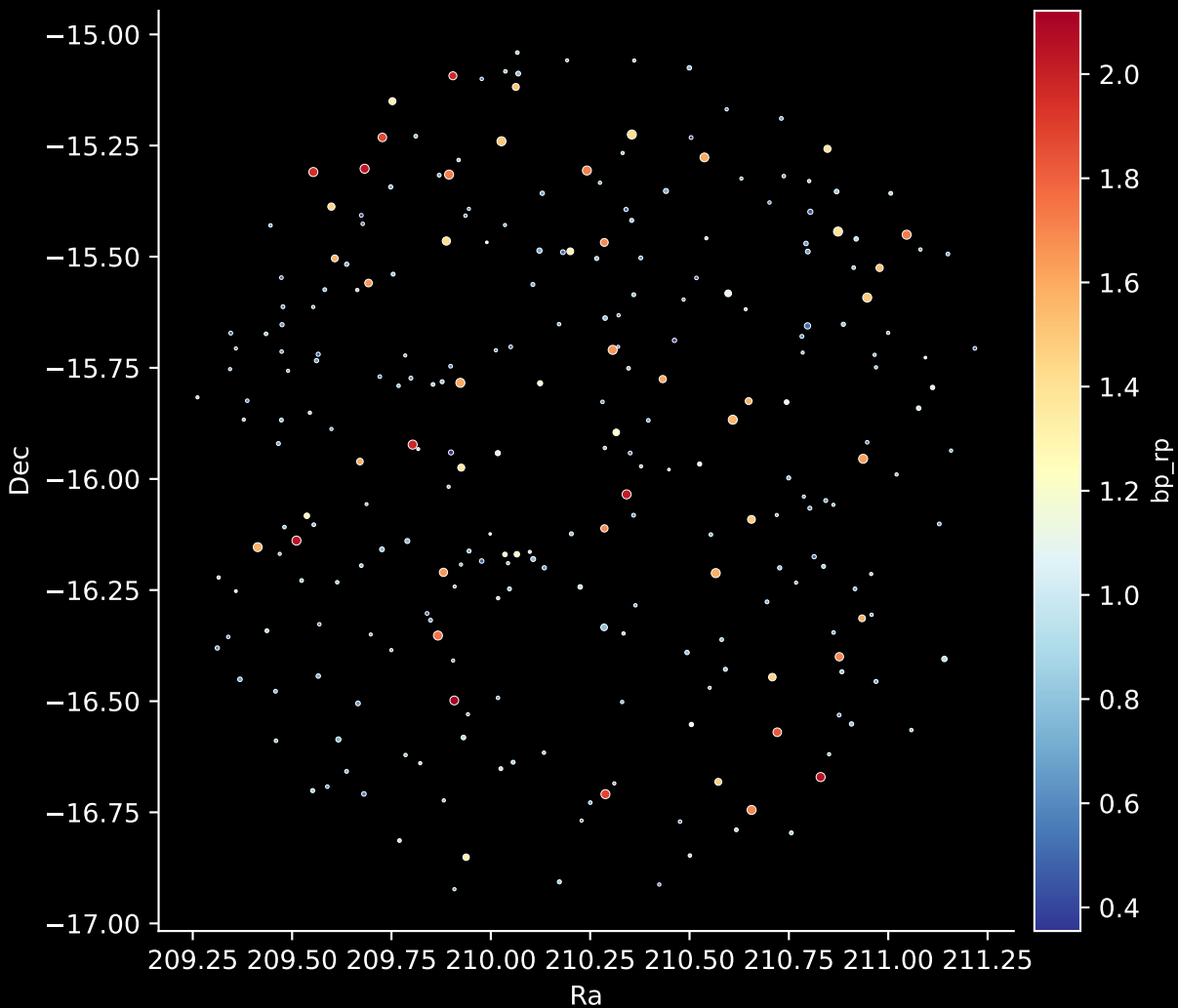
GALAH DR4 Field: [8686] Stars: 266
