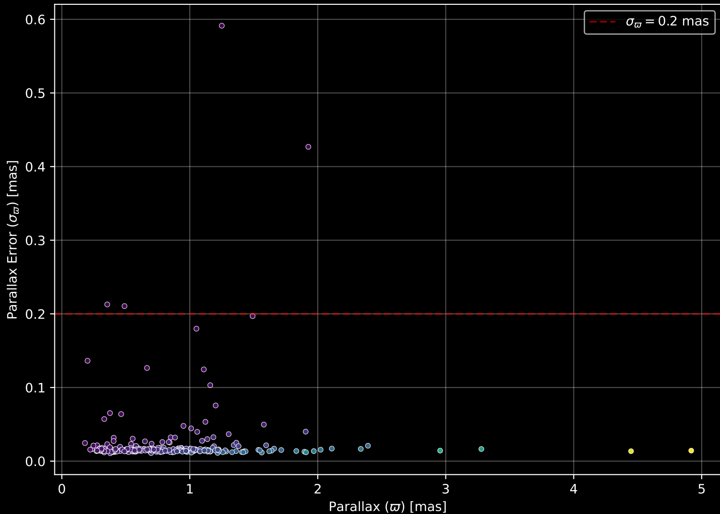
GALAH DR4 Field: [8686] Parallax Quality (n= 266)
